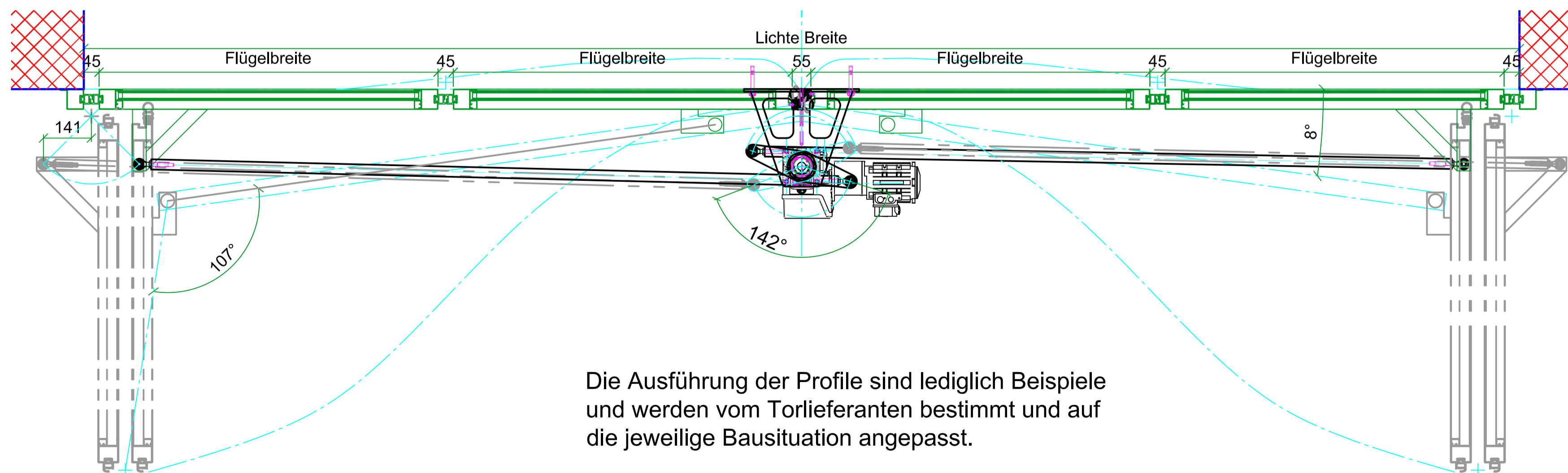
Schnitt D - D
