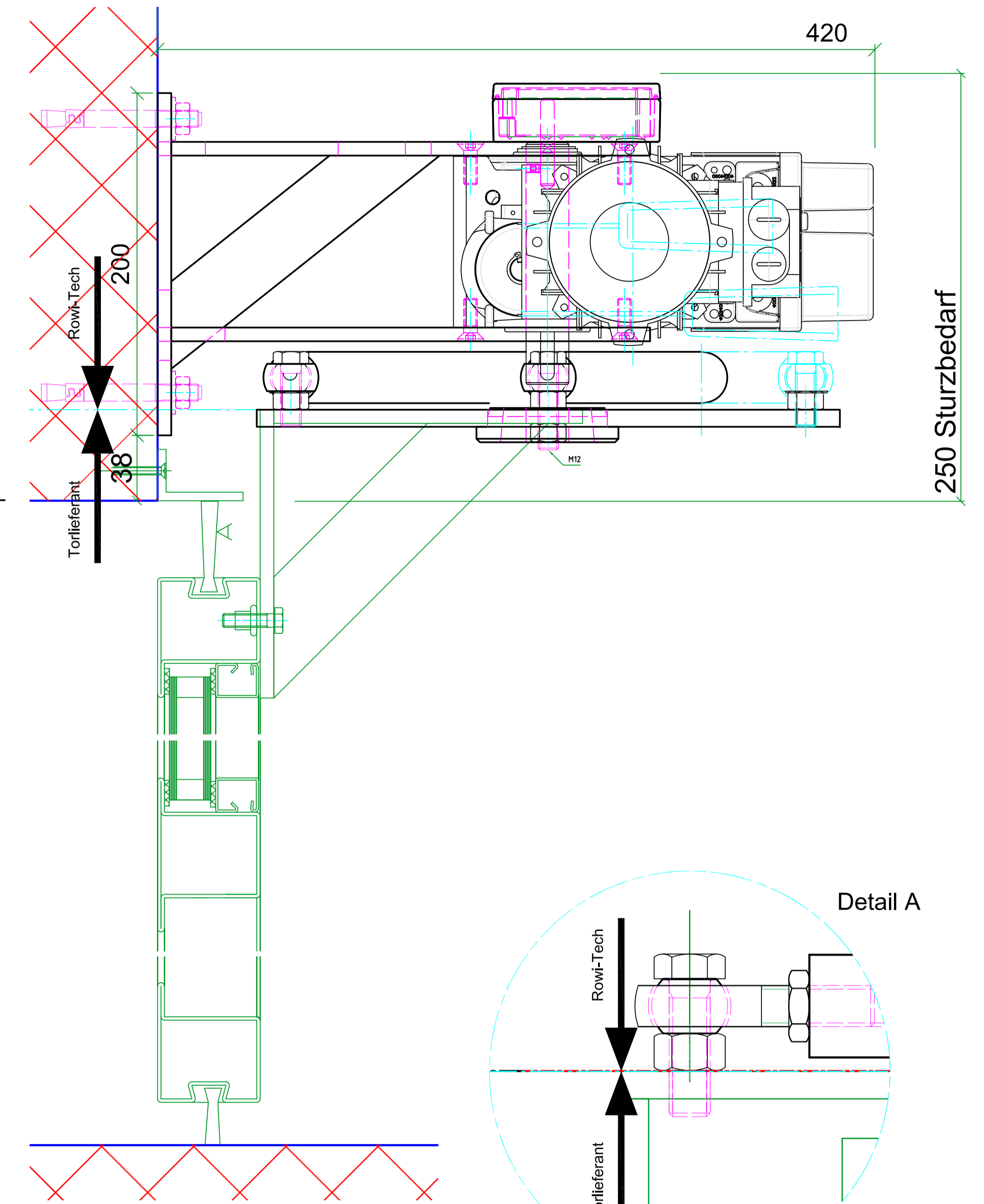
Schnitt A - A
