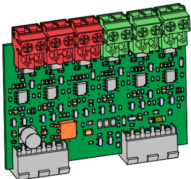
Abb./Fig. 1: TST SURA-6 mit 8,2 kΩ Abschlusswiderstand/TST SURA-6 with 8.2 kΩ resistor/TST SURA-6 avec résistance terminale 8.2 kΩ
