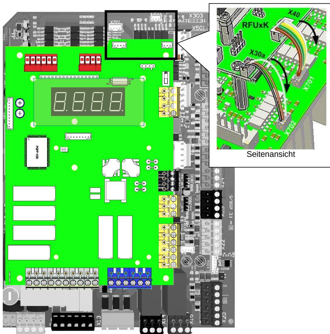
Abbildung 31: TST RFUxK Erweiterungskarte
