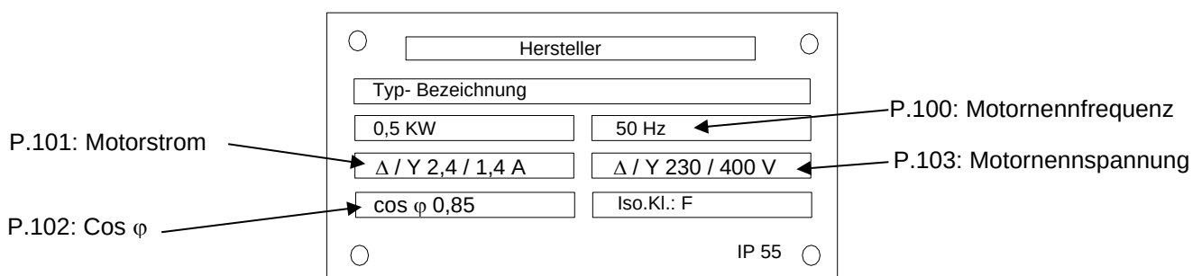
Abbildung 37: Beispiel Motortypenschild (Abb. ähnlich)
