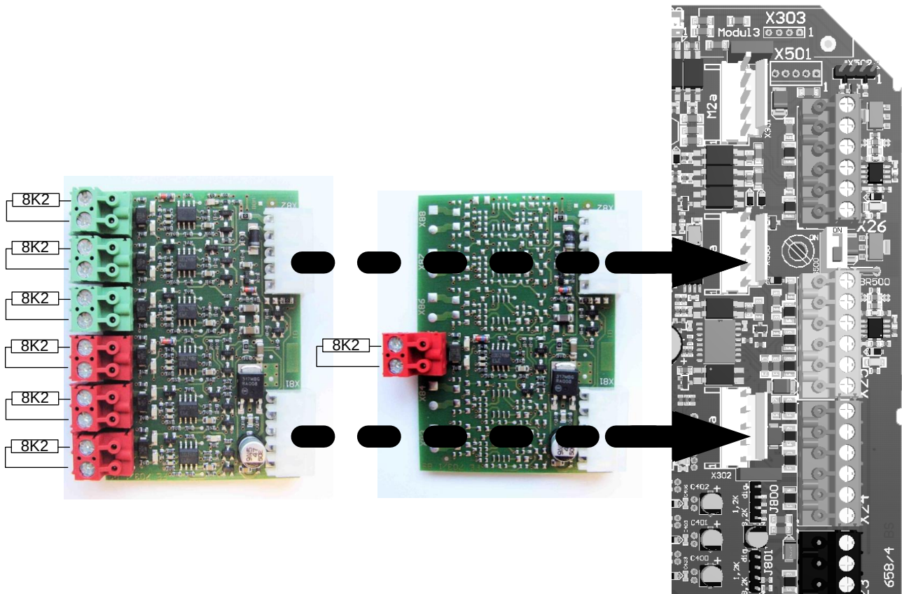
Abbildung 30: Sicherheitsleistenauswerter
