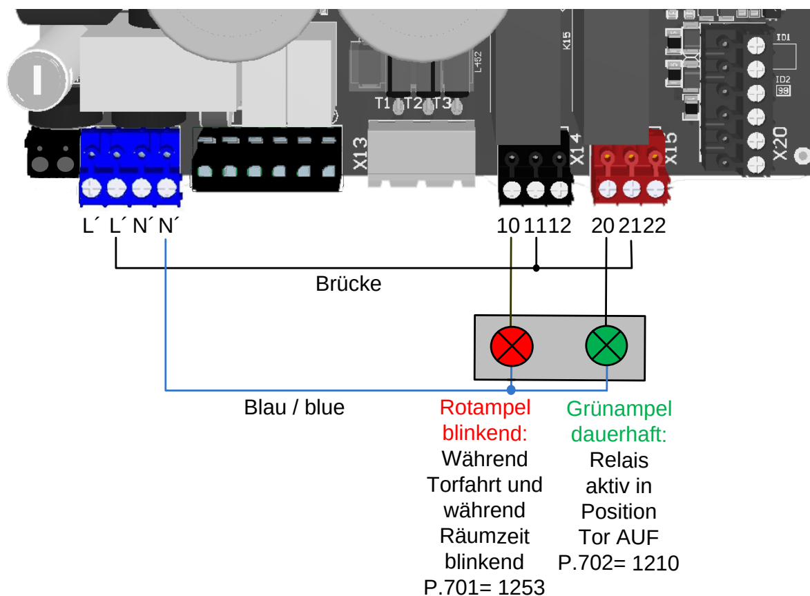
Abbildung 24: Ampelanschluss
