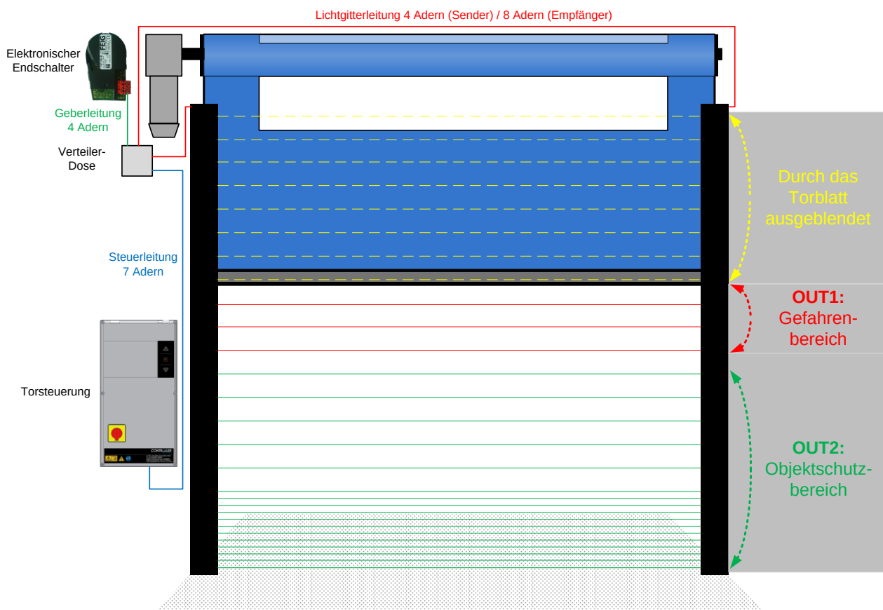
Abbildung 16: Montage des TST LGB
