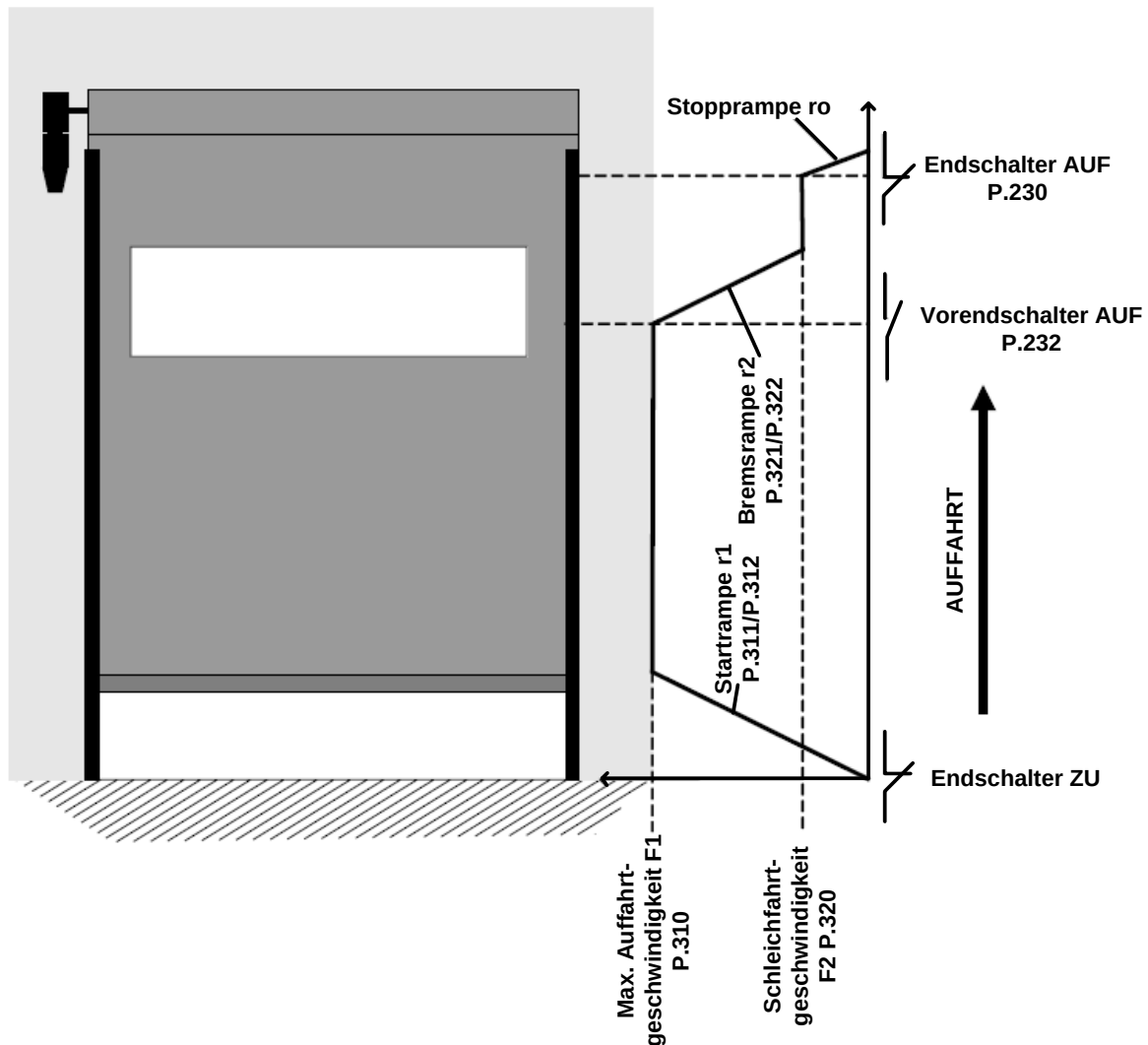
Abbildung 39: Auffahrt mit Frequenzumrichter
