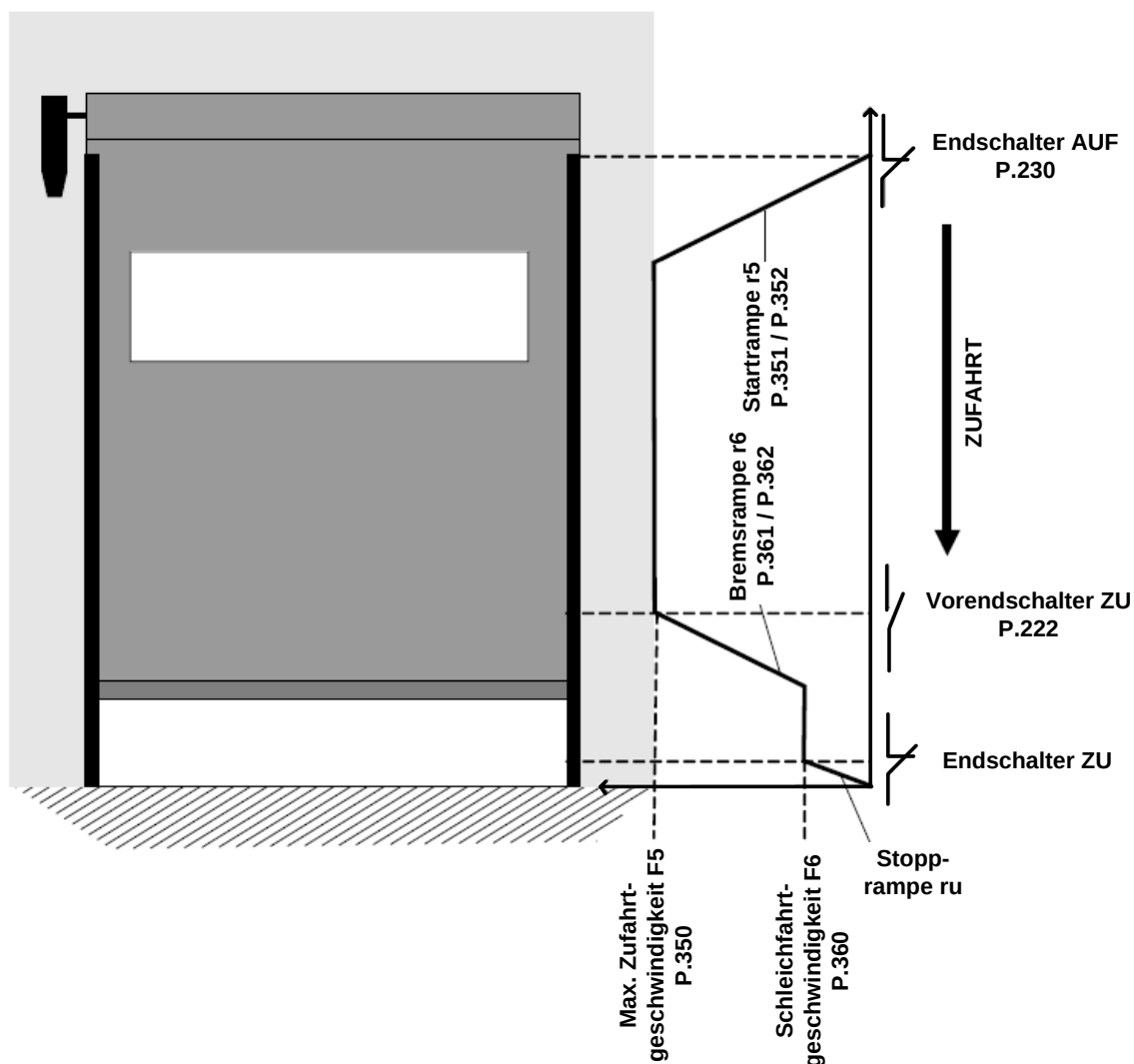
Abbildung 40: Zufahrt mit Frequenzumrichter
