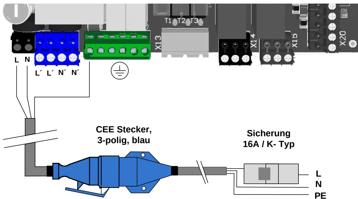
Abbildung 8: Anschluss Netzleitung
