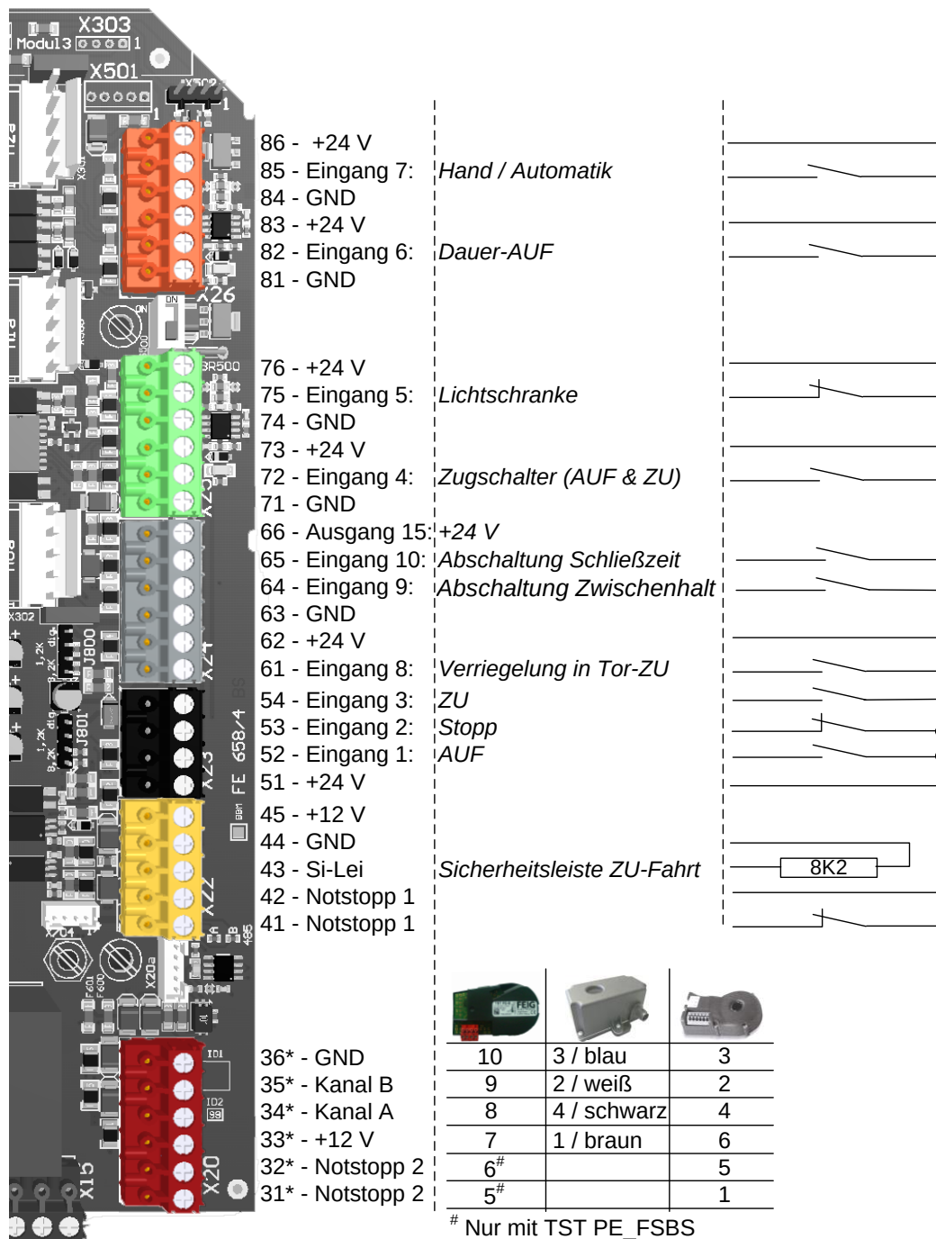
Abbildung 26: Übersicht Eingänge
