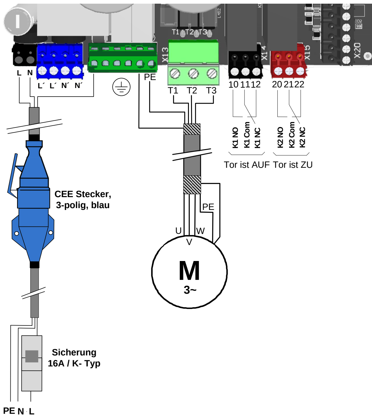
Abbildung 25: Übersicht Ausgänge
