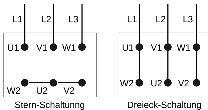
Abbildung 38: Stern- / Dreieckschaltung
