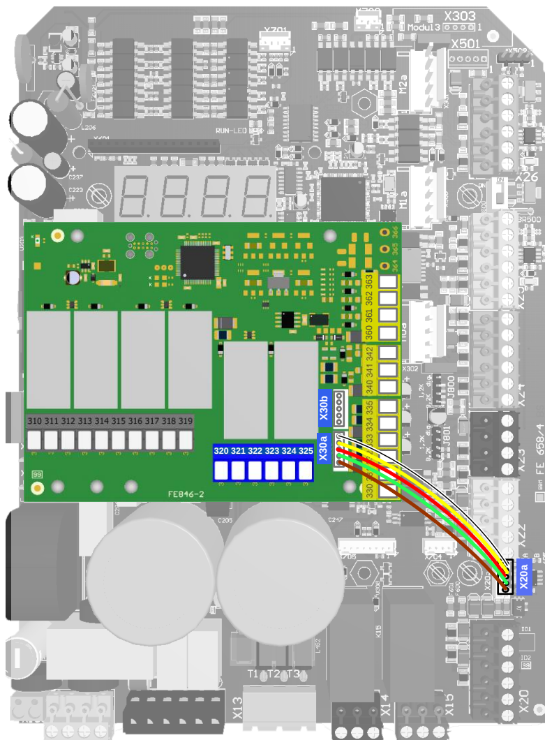
Abbildung 34: Anschlussbeispiel mit der TST RFUxIO-E
