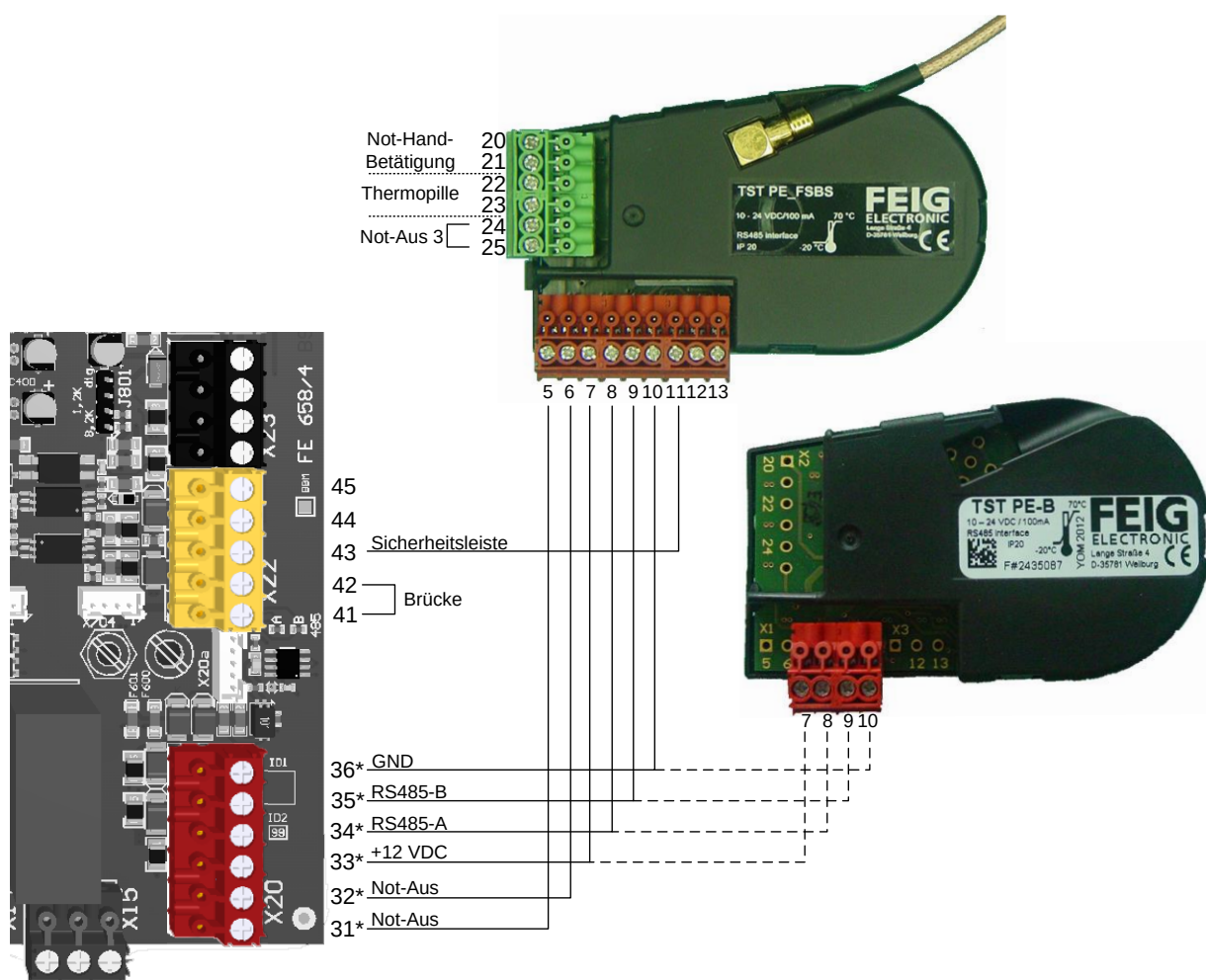
Abbildung 18: Absolutwertgeber TST PE / TST PE FSB
