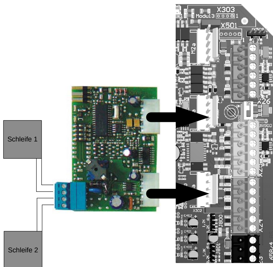
Abbildung 28: Detektorkarte
