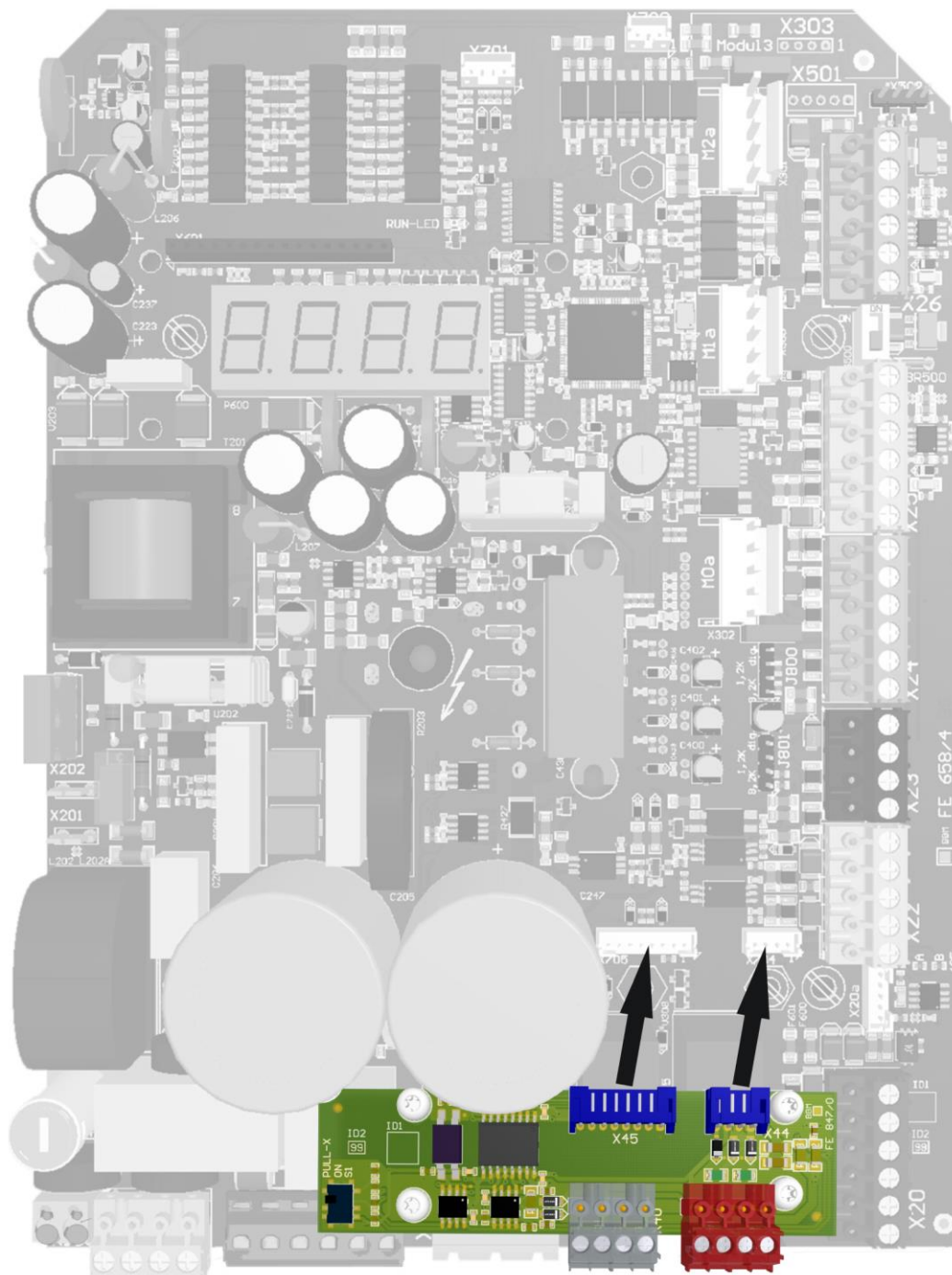
Abbildung 32: Interfacekarte TST RFUxFCOM
