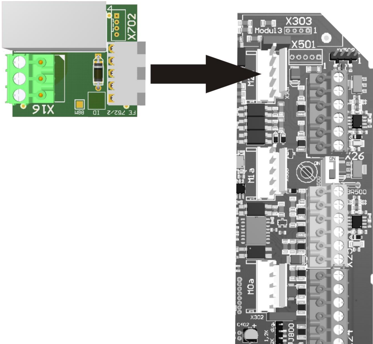
Abbildung 33: Zusatzrelais TST SRA
