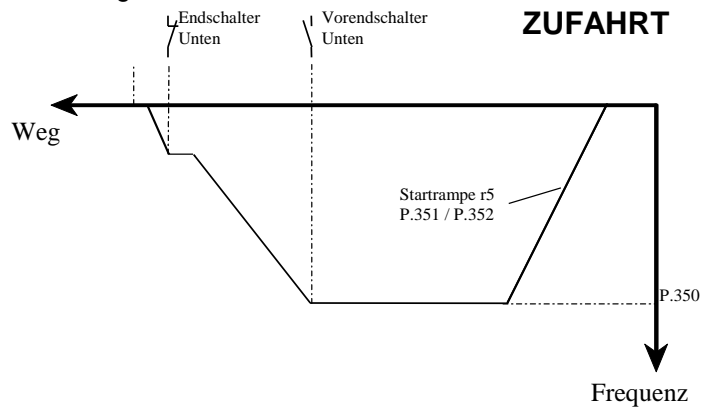
Abbildung 5 Startrampe ZU-Fahrt
