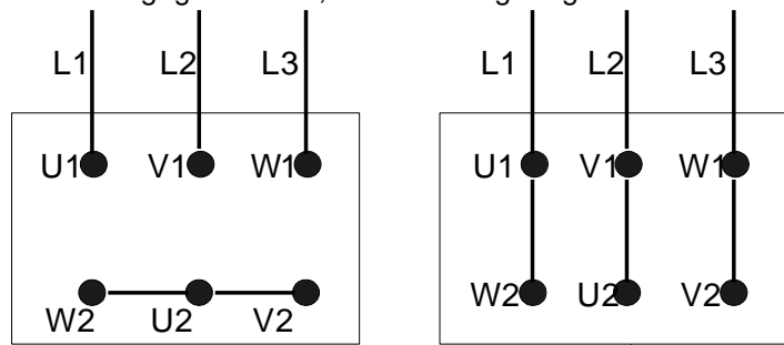
Stern-Schaltung Dreieck-Schaltung
