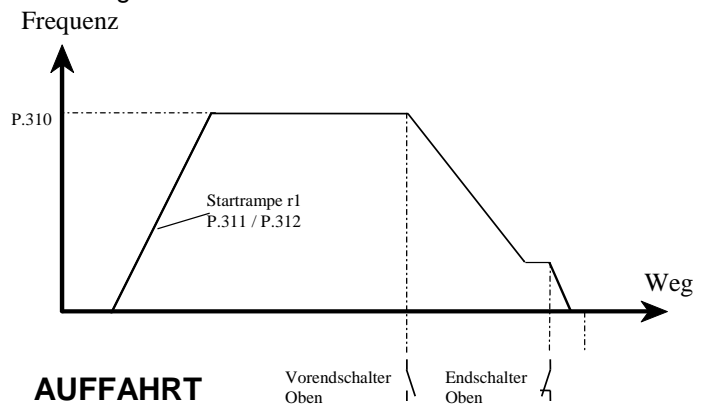
Abbildung 8 Startrampe AUF-Fahrt
