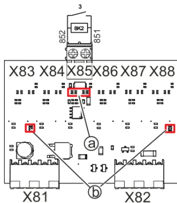
Abb./Fig. 2: Beschreibung der Anschlüsse und LEDs/ Description of connections and LEDs/Description des connexions et des LEDs
