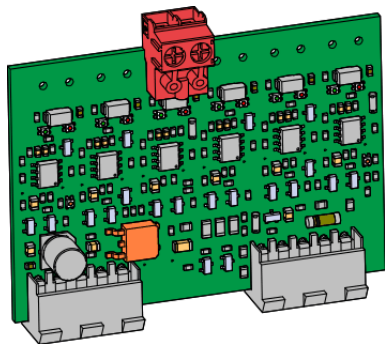
Abb./Fig. 1: TST SURA-1 mit 8,2 kΩ Abschlusswiderstand/TST SURA-1 with 8.2 kΩ resistor/TST SURA-1 avec résistance terminale 8.2 kΩ
